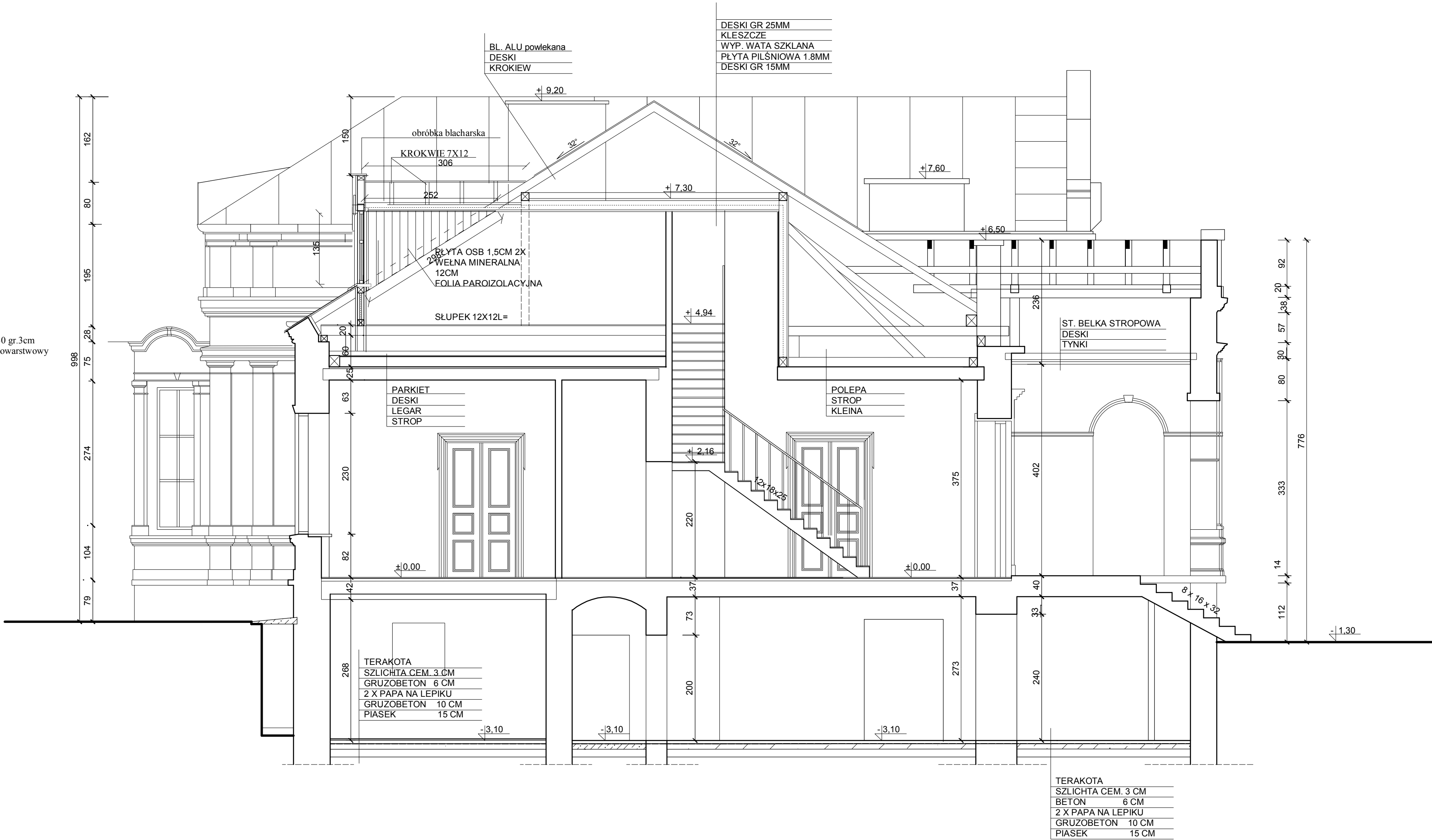
PRZEKRÓJ A -A 1: 50
